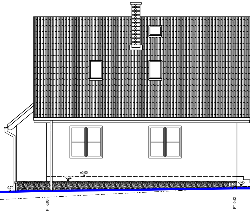
POHLED SEVEROZÁPADNÍ
