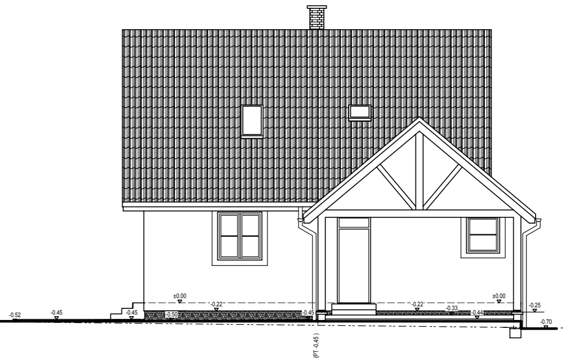
POHLED JIHOVÝCHODNÍ
